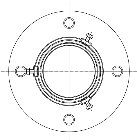
底面図
