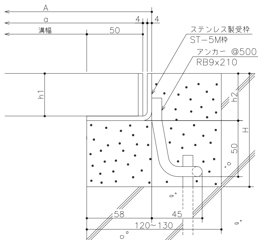
断面詳細図
