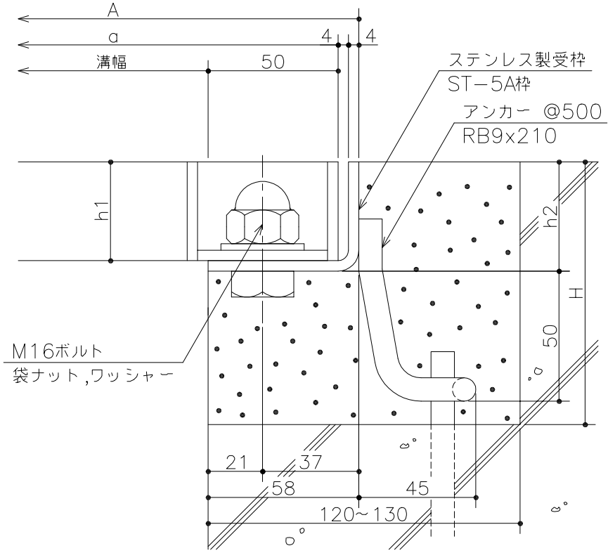
断面詳細図
