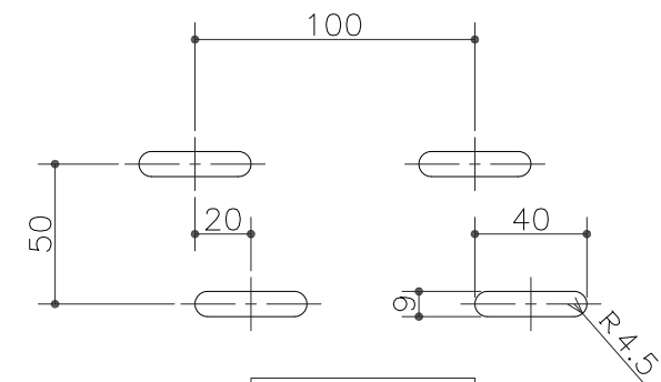
排水穴形状
