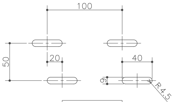
排水穴形状
