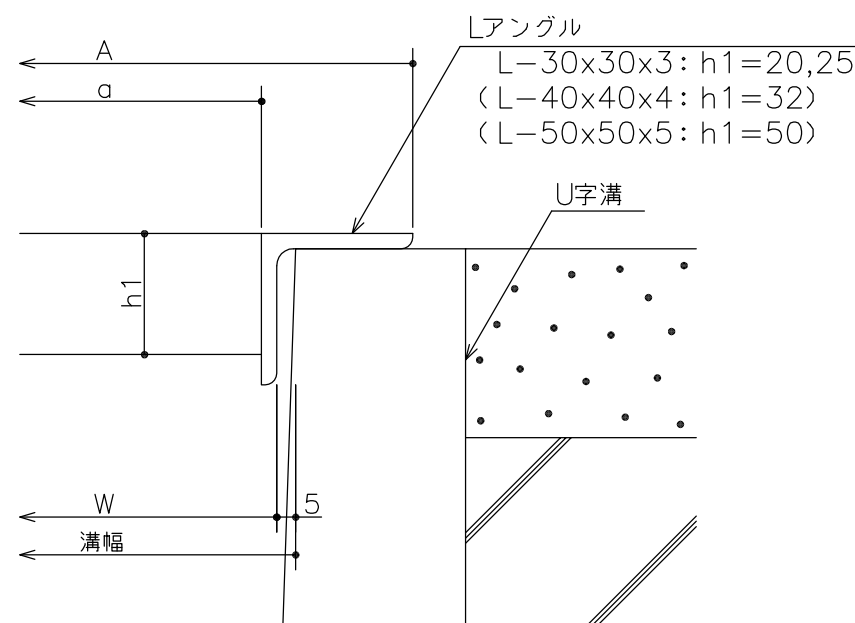
断面詳細図
