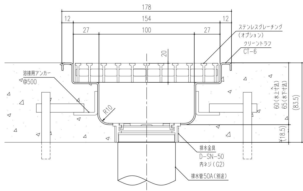
詳細図 S=1/3
