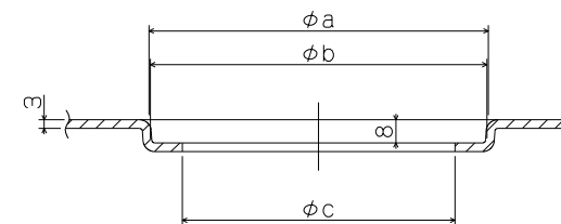
排水金具取付部寸法図
