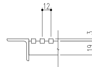
A部 詳細図 S=1/3
