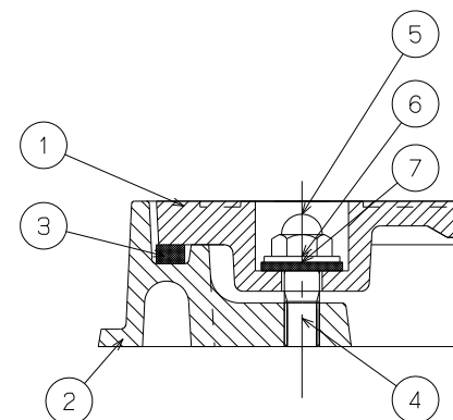
C部詳細
