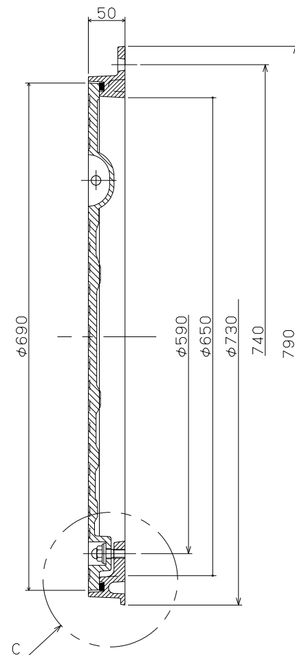
A-B断面図
