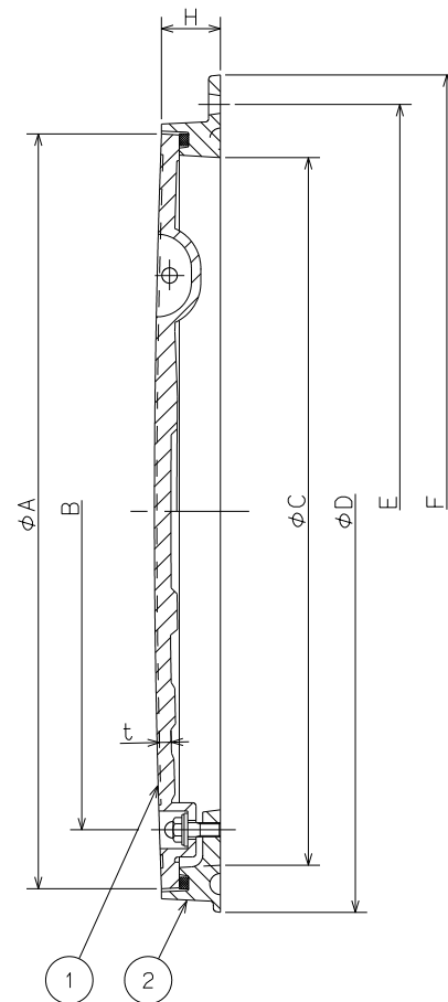
A-O-B断面図
