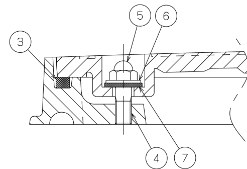
ボルト固定部詳細
