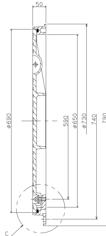
A-O-B断面図
