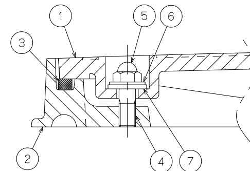
ボルト固定部詳細
