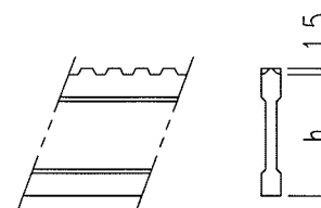
ベアリングバー 詳細図
