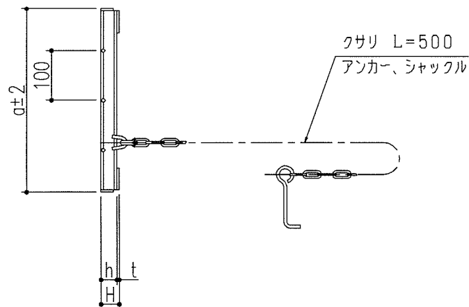
ベアリングバー 詳細図
