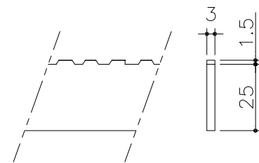
ベアリングバー詳細図
