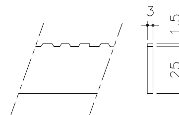
ベアリングバー詳細図
