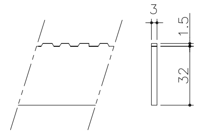
ベアリングバー詳細図
