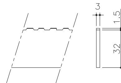
ベアリングバー詳細図
