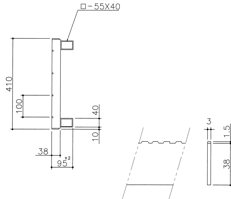
ベアリングバー詳細図
