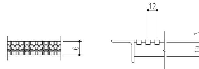
角鋼平面模様 詳細図 S=1/1
