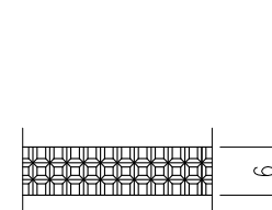
角鋼平面模様 詳細図 S=1/1
