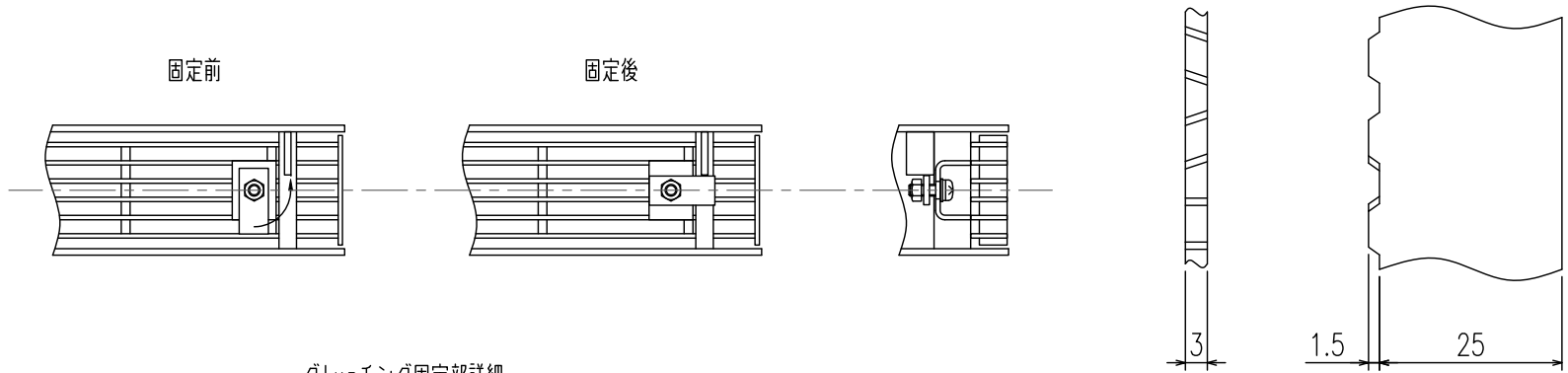
グレーチング固定部詳細
