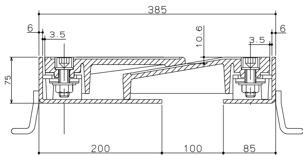
標準時 S=1:3
