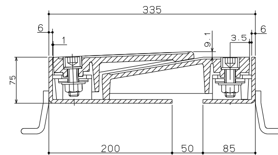
最小可動時 S=1:3
