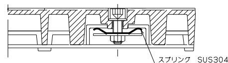
スプリング詳細図 S=1/3
