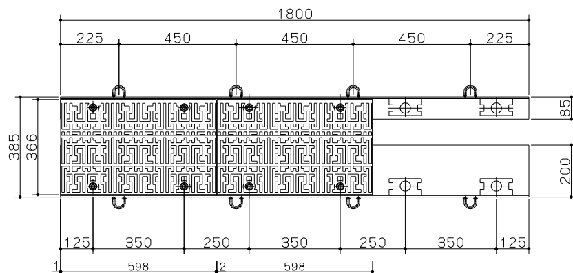
平面図 S=1:10
