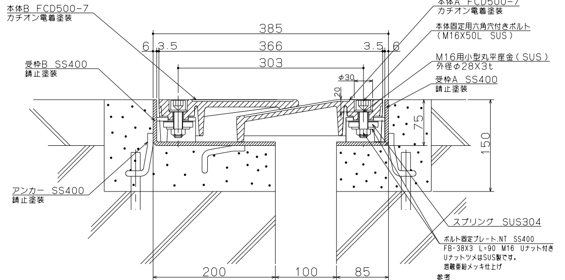
施工断面詳細図 S=1:3
