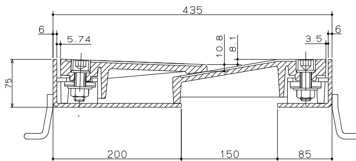
最大可動時 S=1:3
