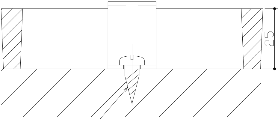
タッピンネジM6×14 (別途)
