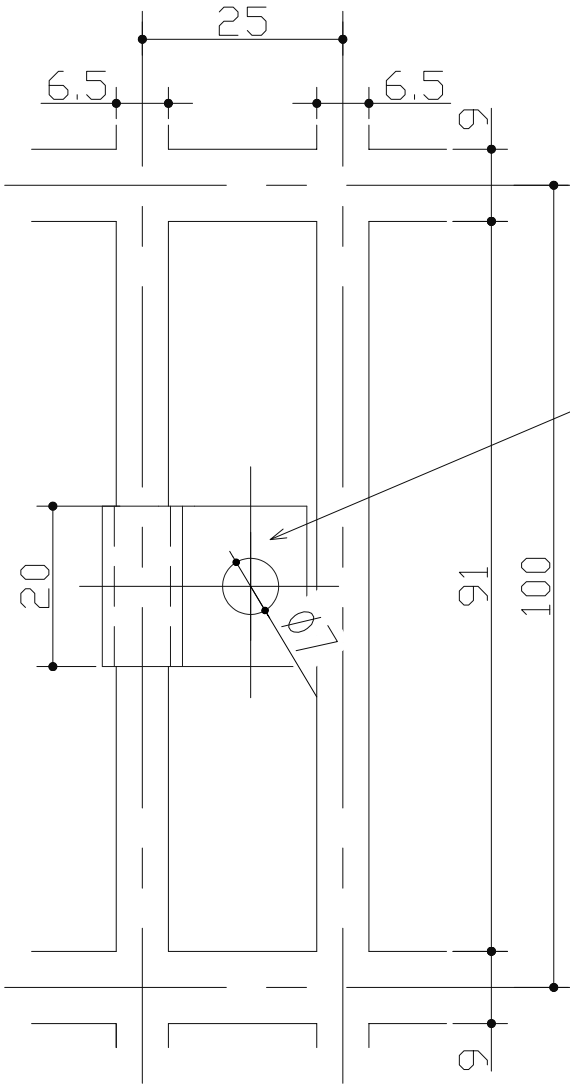
取付金具 25L
