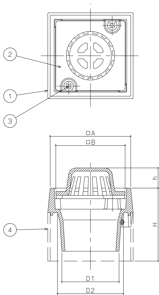
A-A断面図
