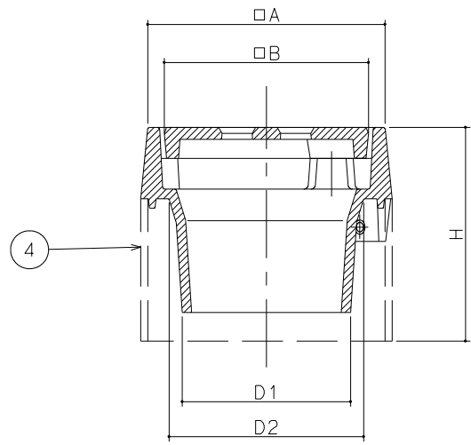
A-A断面図
