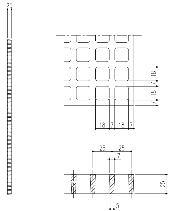
詳細図S=1/2
