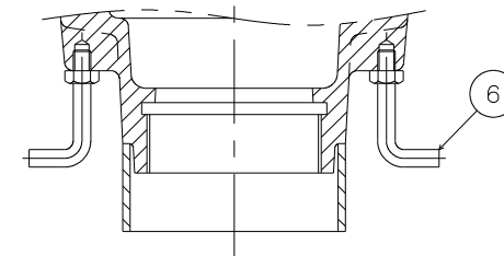
呼称50スリーブ装着図
