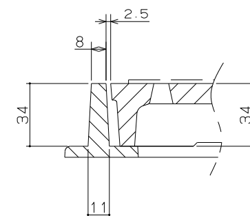
受枠とふた 嵌合部詳細図
