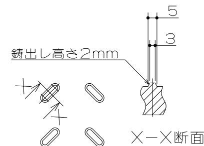
滑り止め模様詳細図
