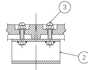
固定部断面
