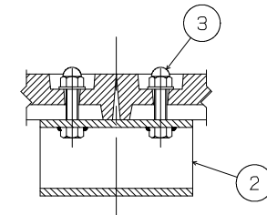
固定部断面
