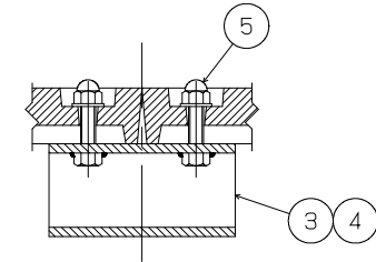
固定部断面
