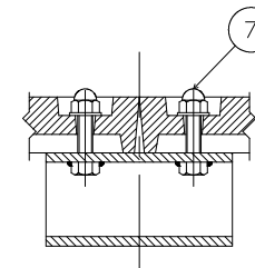
固定部断面
