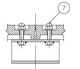
固定部断面
