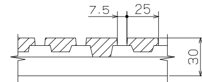
細目断面
