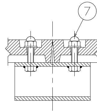
固定部断面
