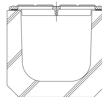
U字溝納まり図
