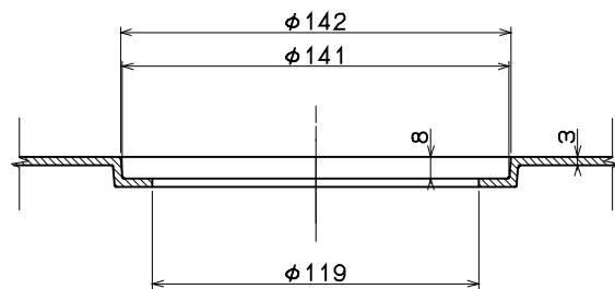
防水パン穴寸法
