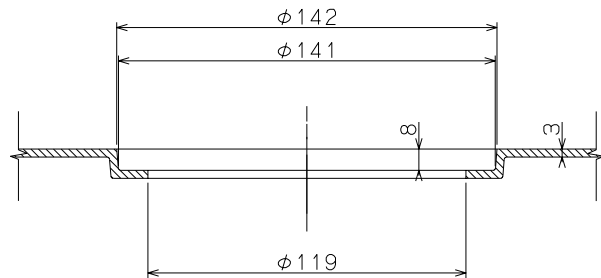
防水パン穴寸法
