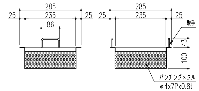
ストレーナー詳細図
