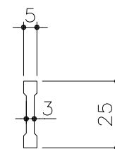
ベアリングバー-詳細図
