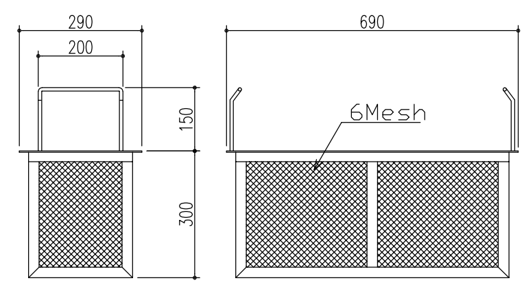
ストレーナー詳細図
