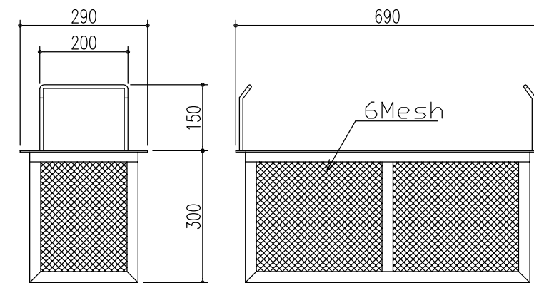
ストレーナー詳細図
