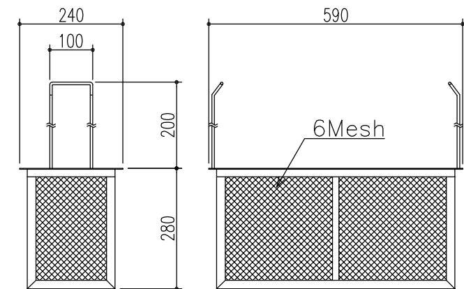
ストレーナー詳細図
