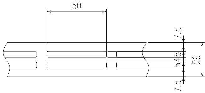
排水部拡大詳細図
