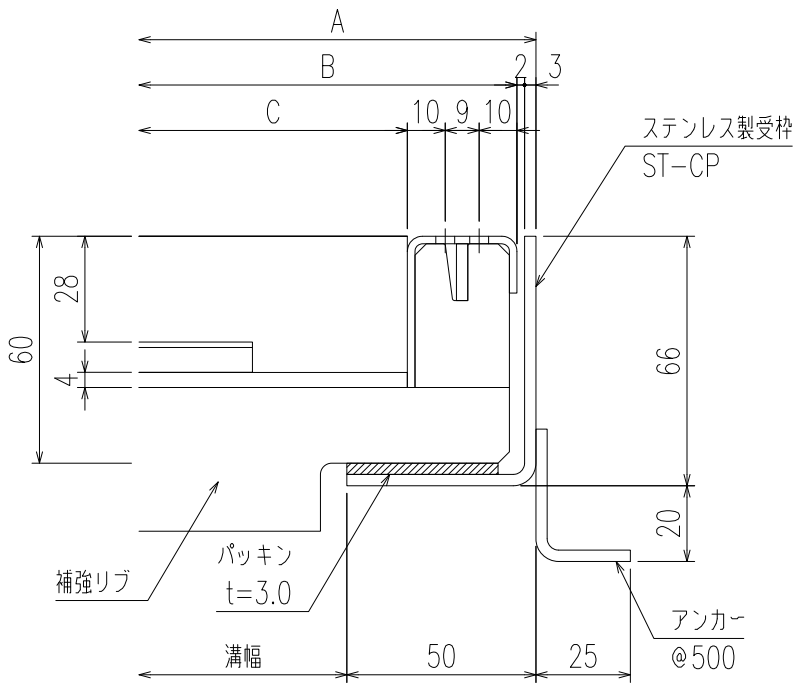
断面拡大詳細図
