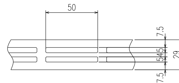
排水部拡大詳細図
