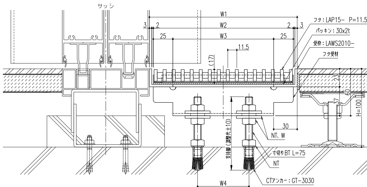
断面詳細図 (参考納まり図) S=1/2
