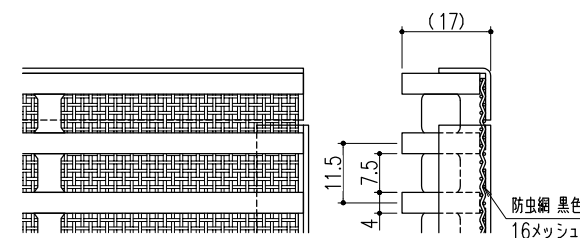
フタ詳細図 S=1/1
