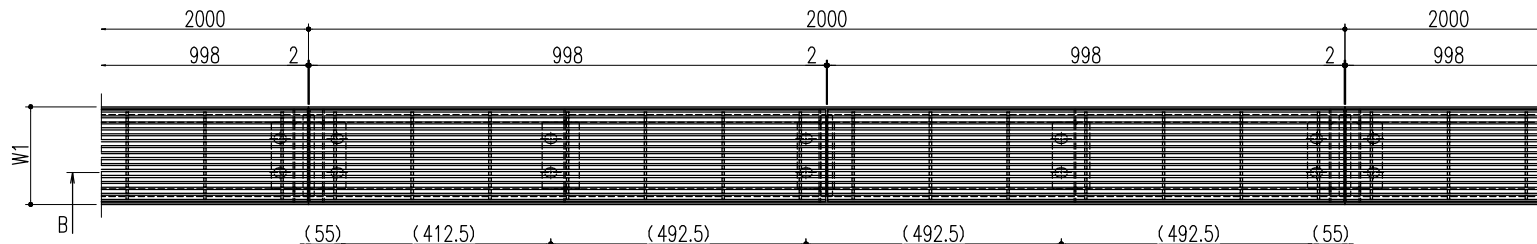
平面詳細図 S=1/10
