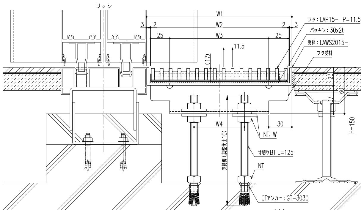
断面詳細図 (参考納まり図) S=1/2
