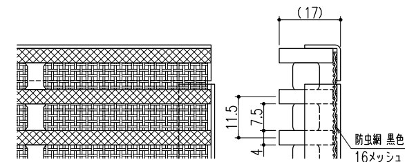
フタ詳細図 S=1/1
