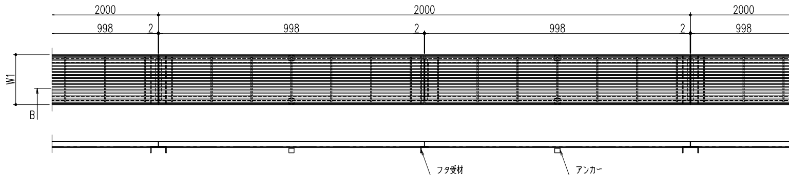
平面詳細図 S=1/10
