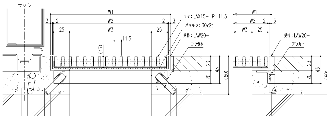
断面詳細図(参考納まり図) S=1/2
