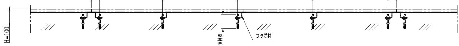
矢視B受枠断面図 S=1/10
